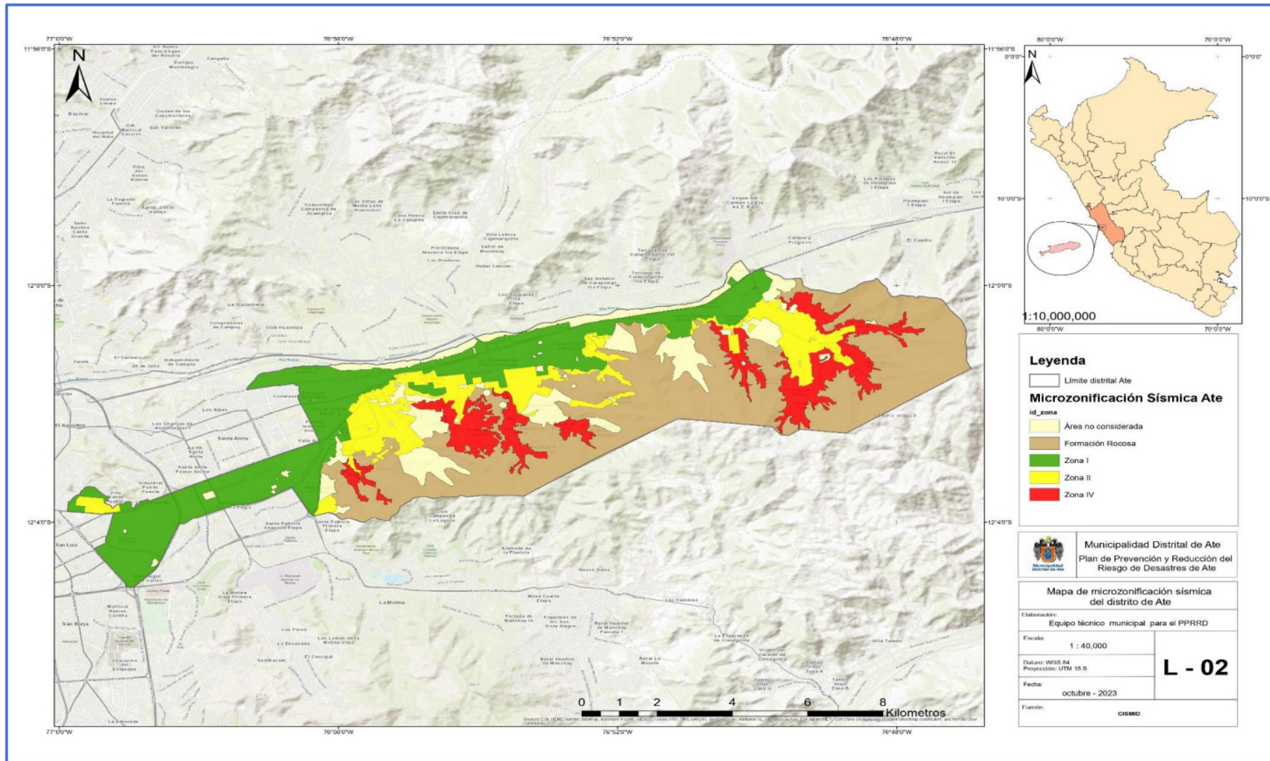
Figura N° 31 - Mapa de Microzonificación Sísmica del Distrito de Ate.
